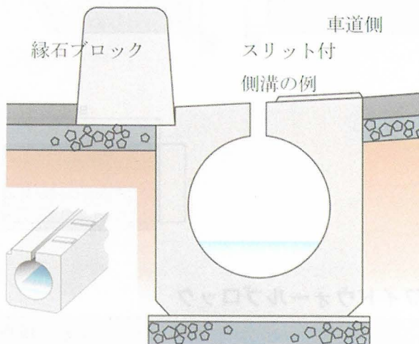
● 円形型スリット付側溝の施工断面例
